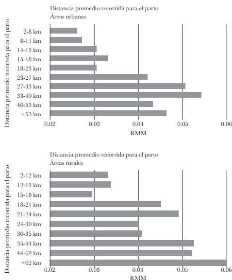
Gráfica 5 Relación entre distancia promedio a clínica resolutive y RMM
